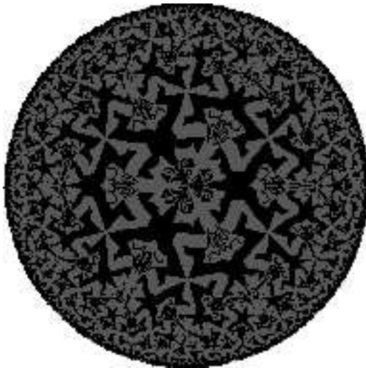
Fig. 5.8. Pattern 53
