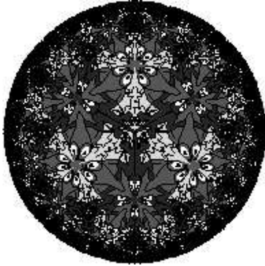
Fig. 5.10. Pattern 85
